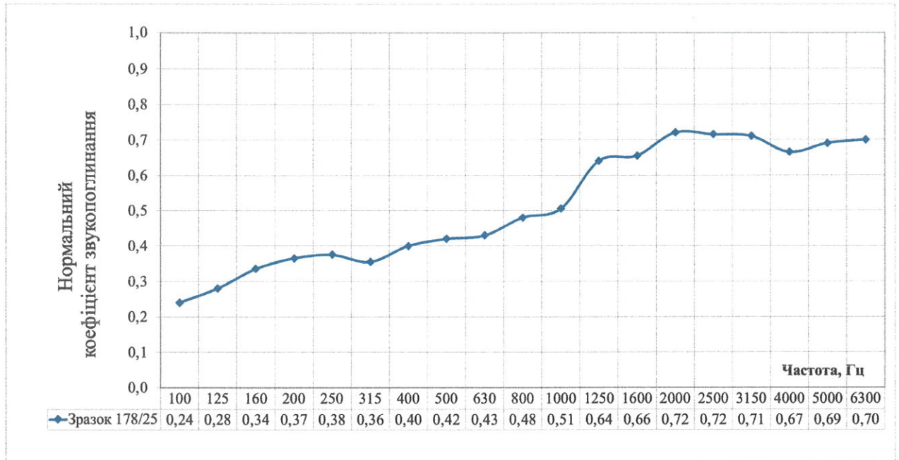
Рисунок 1 - Частотна характеристика нормального коефіцієнта звукопоглинання мінераловатних плит на синтетичному зв'язуючому марки «НТ Покрівля 180» виробництва ТОВ «НОВОТЕРМ» завтовшки 50 мм та густиною 180 кг/м 3
