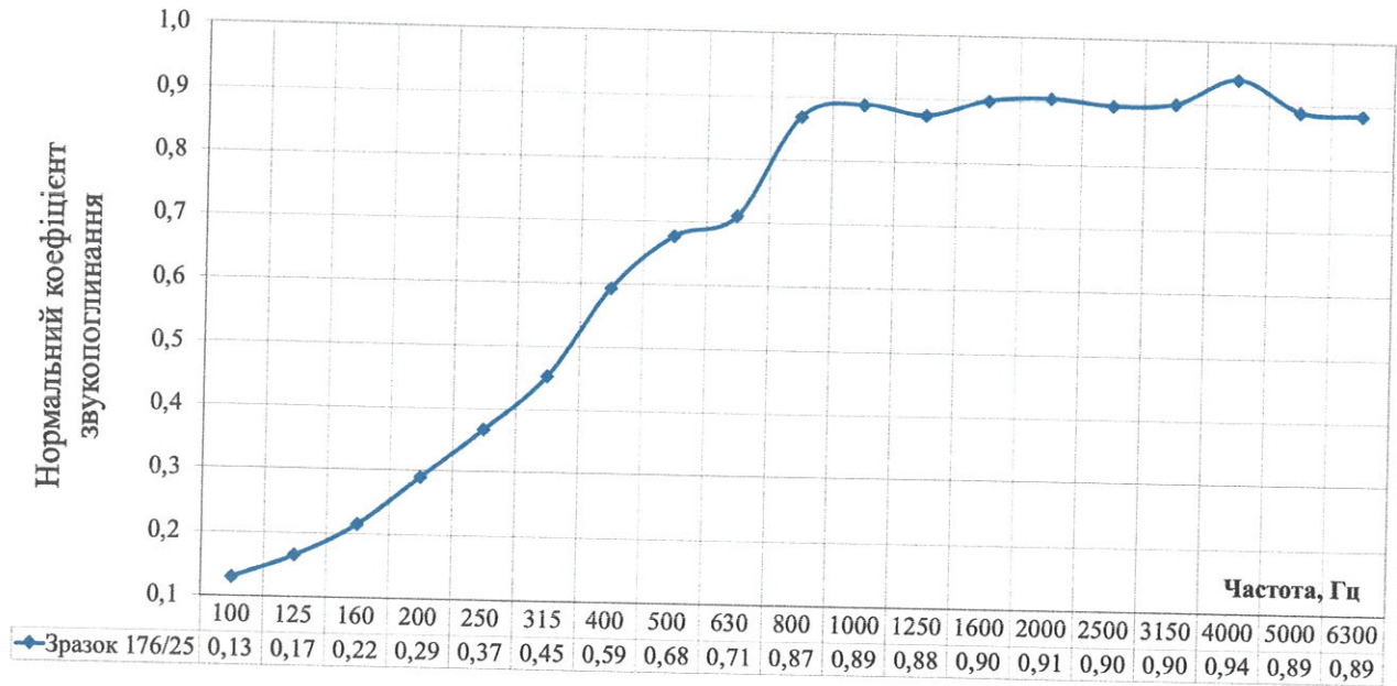
Рисунк 1 - Частотна характеристика нормального коефіцієнта звукопоглинання мінераловатних плит на синтетичному зв'язуючому марки «NT FasPRO 7,5» виробництва ТОВ «НОВОТЕРМ» завтовшки 50 мм та густиною 80 кг/м 3
