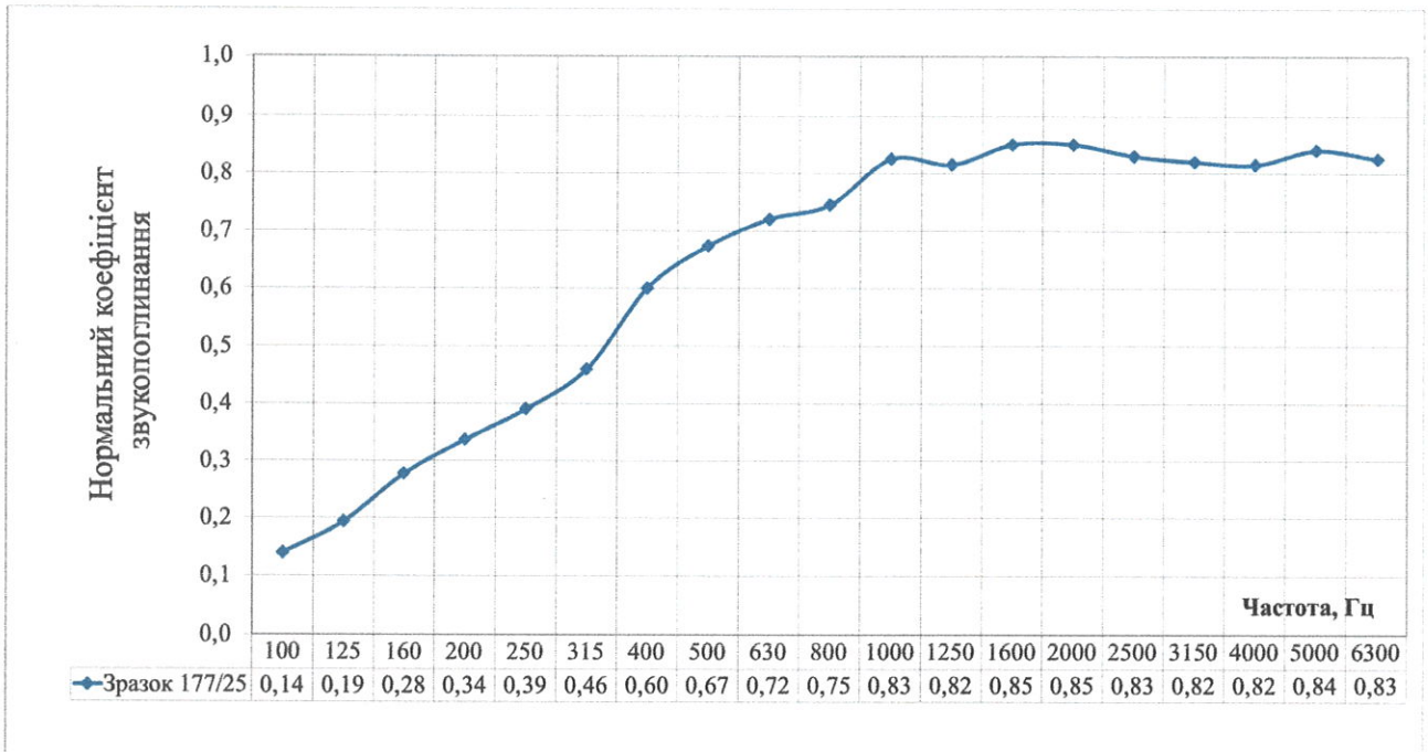
Рисунок 1 - Частотна характеристика нормального коефіцієнта звукопоглинання мінераловатних плит на синтетичному зв'язуючому марки «NT FasPRO 10» виробництва ТОВ «НОВОТЕРМ» завтовшки 50 мм та густиною 95 кг/м 3
