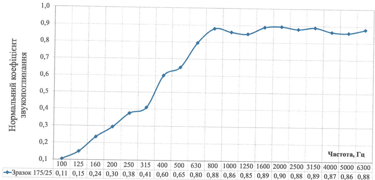
Рисунок 1 - Частотна характеристика нормального коефіцієнта звукопоглинання мінераловатних плит на синтетичному зв'язуючому марки «NT Fasad 7,5» виробництва ТОВ «НОВОТЕРМ» завтовшки 50 мм та густиною 90 кг/м 3
