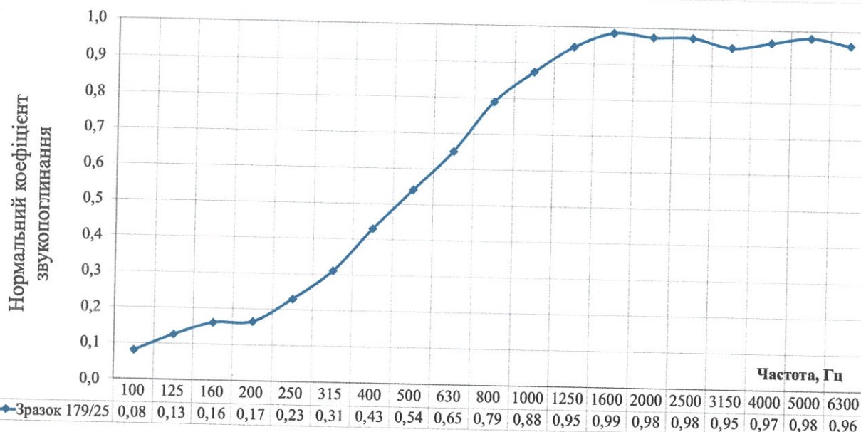
Рисунок 1 - Частотна характеристика нормального коефіцієнта звукопоглинання мінераловатних плит на синтетичному зв'язуючому марки «НТ Лайт 30» виробництва ТОВ «НОВОТЕРМ» завтовшки 50 мм та густиною 30 кг/м 3
